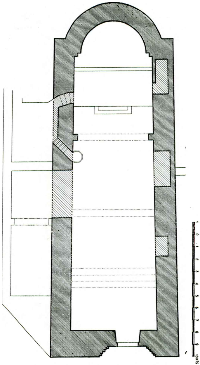
Planta de l'església parroquial de Vinaixa
